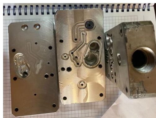
USZKODZONE GŁOWICE
